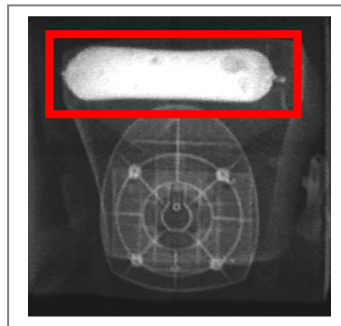
„Backscatter“- Bild mit 1,3 kg Sprengstoff; im Doppel-Energiebild nicht erkennbar !
